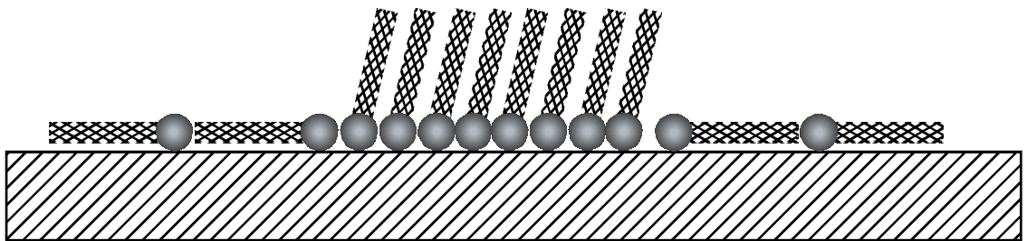
(d) Nucleation of solid phase islands
