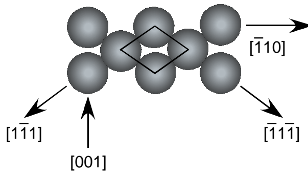
(b) bcc(110)
